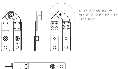
FPQ IOFA - Angle intérieur - extérieur variable
