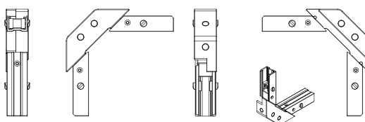
FPQ IF90 - Angle intérieur 90°
