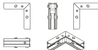
FPQ OF90 - Angle extérieur 90°
