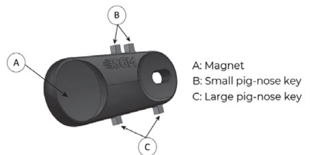
POI Spanner
