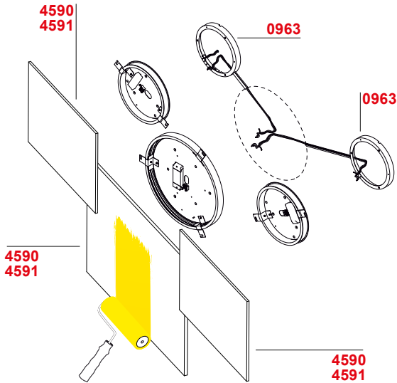
Esempio di installazione multipla con distanziali 0963 Example of multiple installation with spacers 0963
