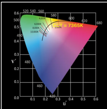
CIE 1976
