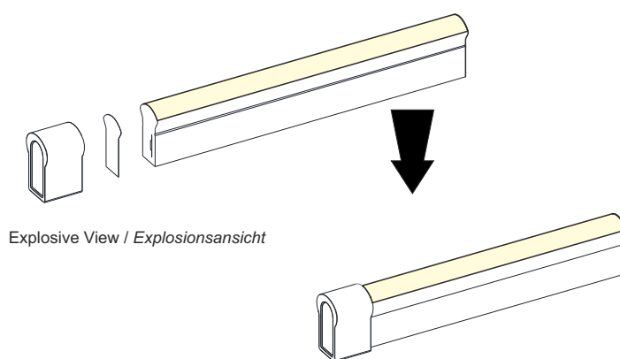
Finished Assembly View / Ansicht zusammengebaut
