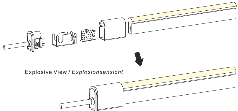
Finished Assembly View / Ansicht zusammengebaut.
